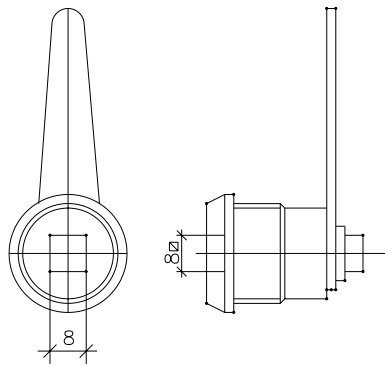
DETALLE CIERRE CUADRADILLO INTERIOR HEMBRA 8 MM
